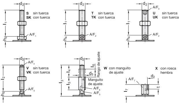
Versiones de vástago roscado
