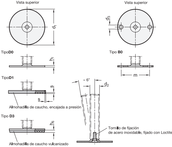
Versiones de vástago roscado
